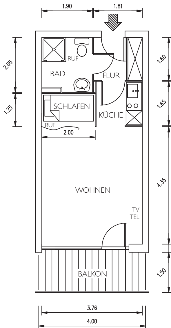
Rohbaumaße in Metern
