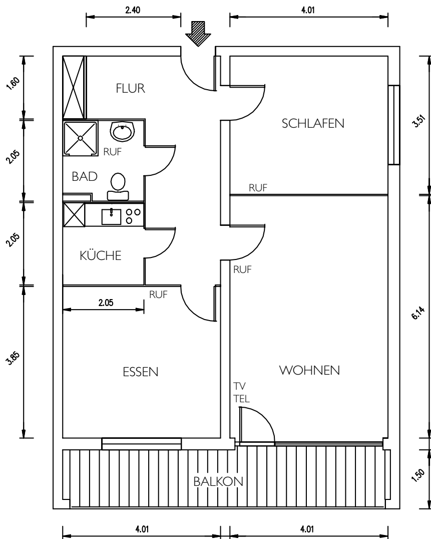
Rohbaumaße in Metern
